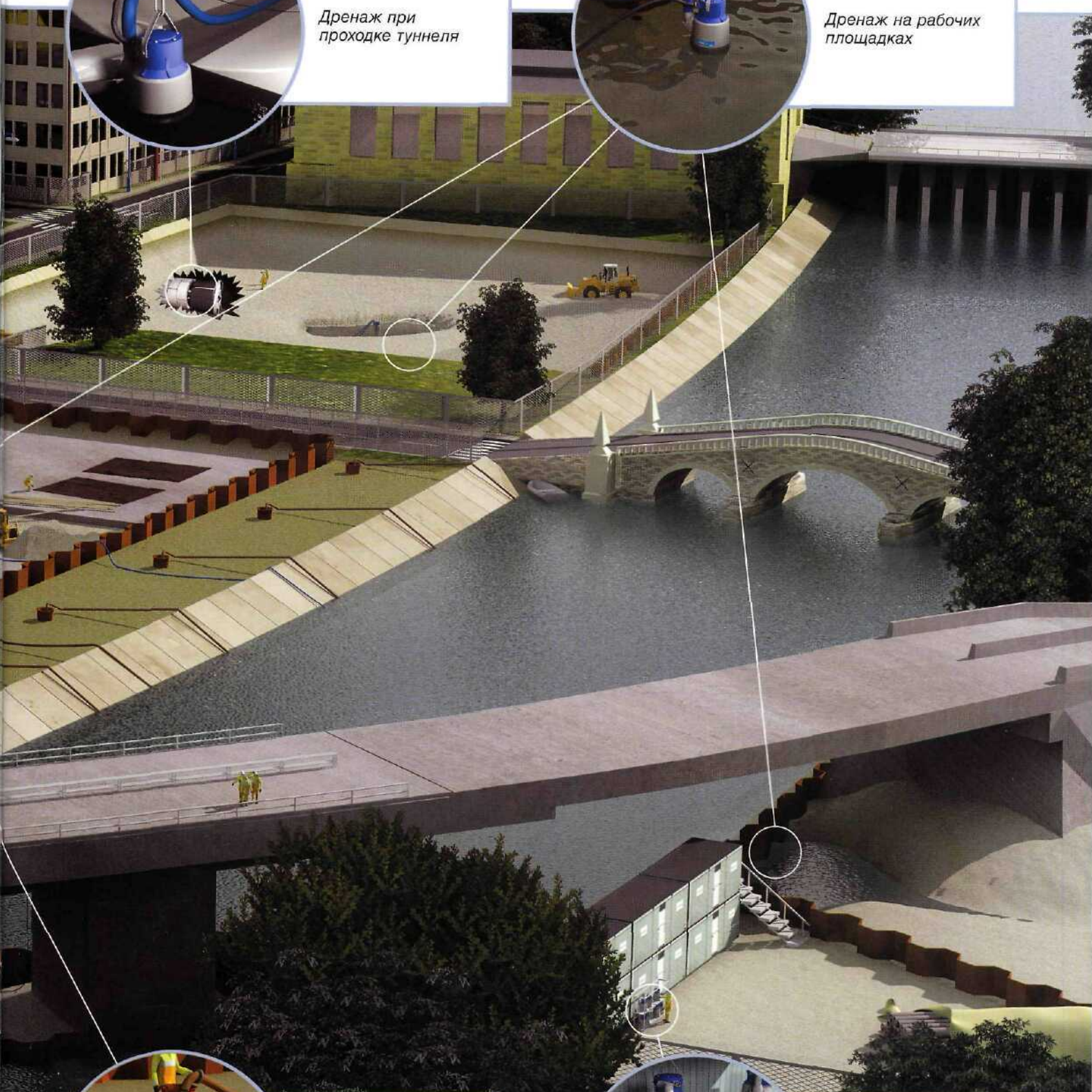
Активный водоотлив с помощью малогабаритных трубопроводных насосов
